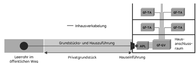
Prinzipiskizze Mehrfamilienhaus
